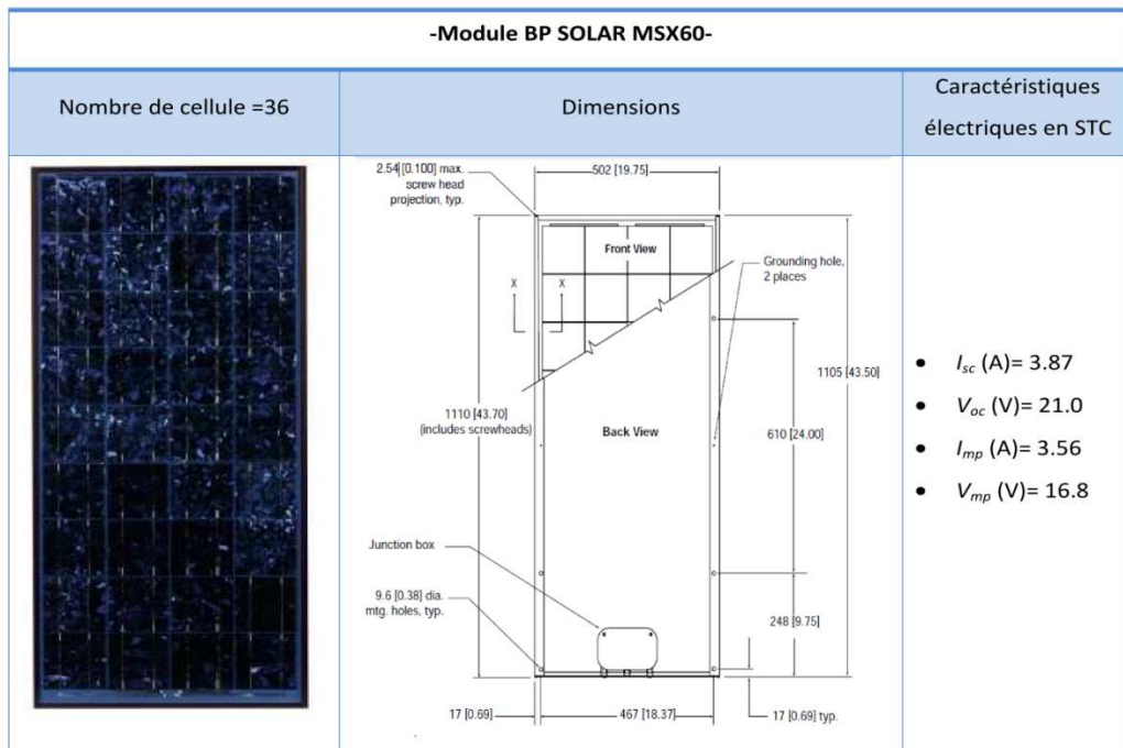
Figure 2.24: Caractéristiques physiques et électrique du Module BP SOLAR MSX60
