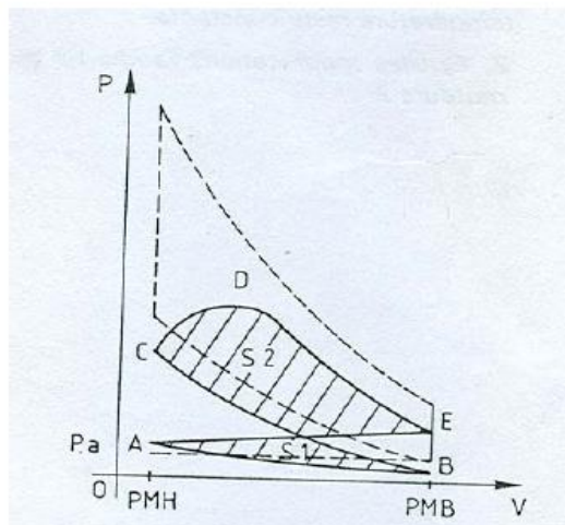
Fig. 3.2 Diagramme réel avant réglage
