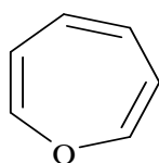
oxepine
