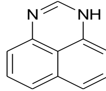
1H-perimidine
