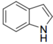
1H-indole
