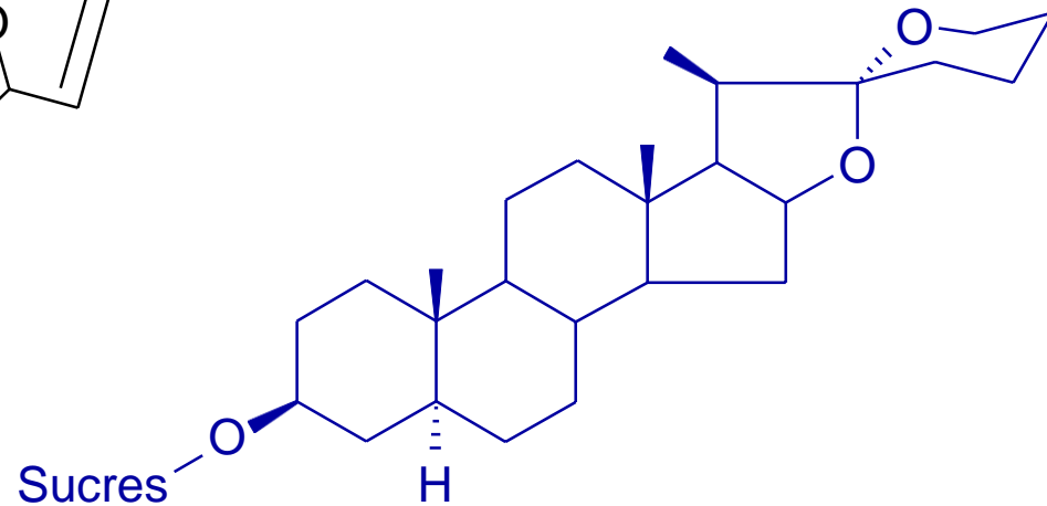
Saponine
