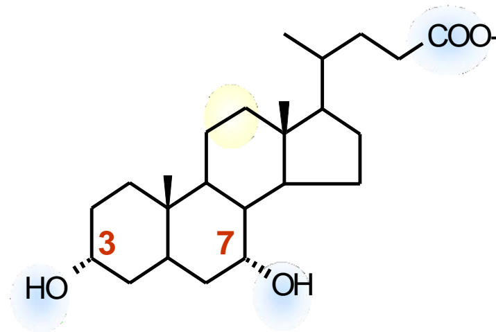
Acide chénodésoxycholique
