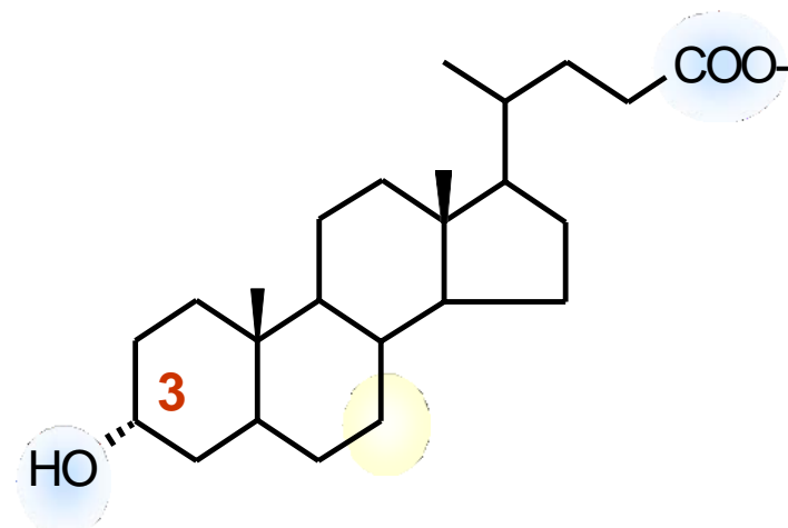
Acide lithocholique
