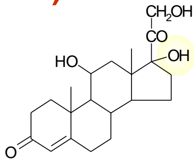
Cortisol (C21)
