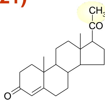
Progestérone (C21)
