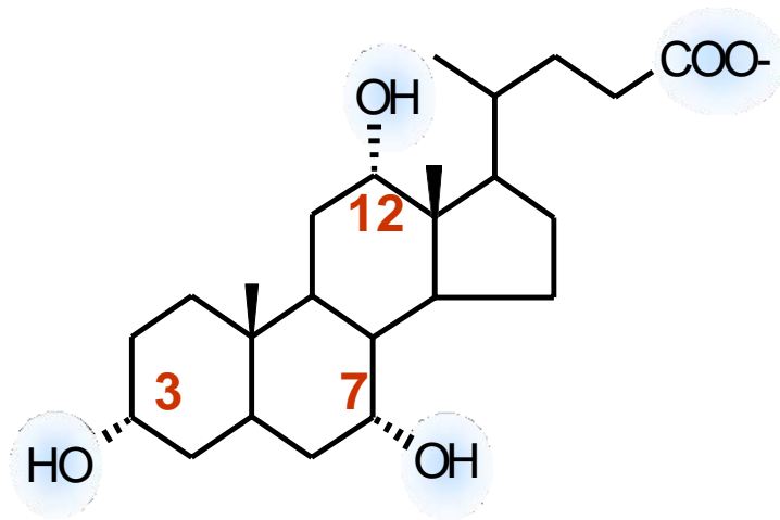
Acide cholique
