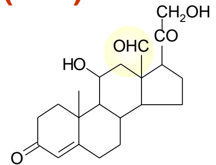
Aldostérone (C21)
