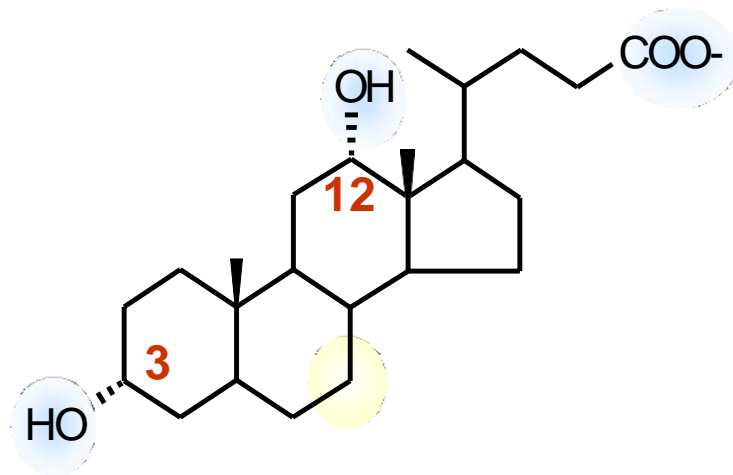
Acide désoxycholique
