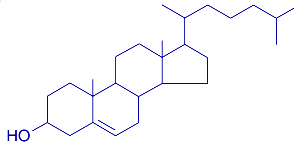
Cholestérol
